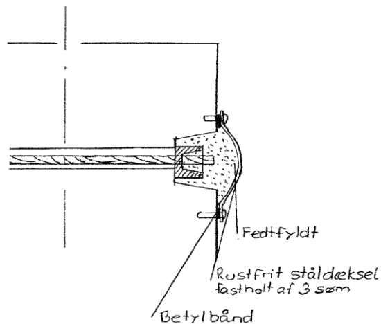
Figur 1. Afdækningen består af en (fedtfyldt) rustfri af-dækning fastgjort på låseklodsens med 3 søm. Hætten tættes via en pakning af betylbånd, som samles med overlæg. Inden fastgørelse affedtes betonen, så betylbånd kan hænge ved og stålhatten klemmes jævnt til be-tonen med hjælp af sømmene.
