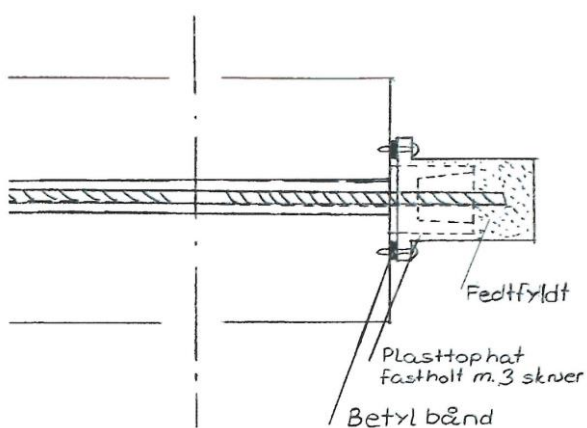
Figur 2. Afdækningen består af en (fedtfyldt) hætte i plast tæt-net via en pakning af betylbånd, som samles med overlæg på hættens. Inden fastgørelse affedtes forankringspladen på trap-petrinet, så betylbåndet kan hænge ved.
