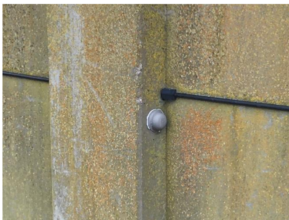
Foto 11. Afdækning på Spæncom beholder i form af plastafdækning sat i fugemasse.
